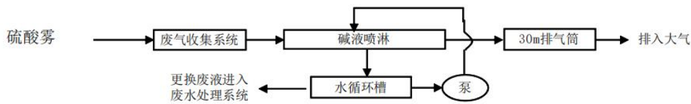
图4-2-1 酸性废气处理流程图
