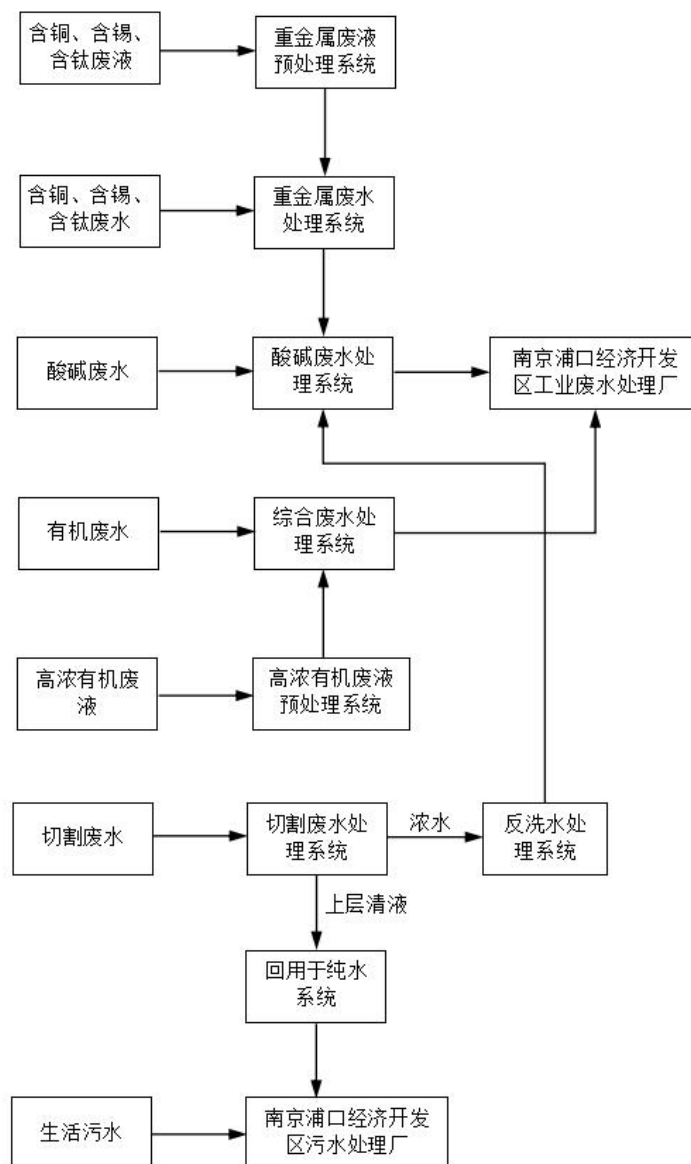
图 4-2-2 本项目废水排放走向图
