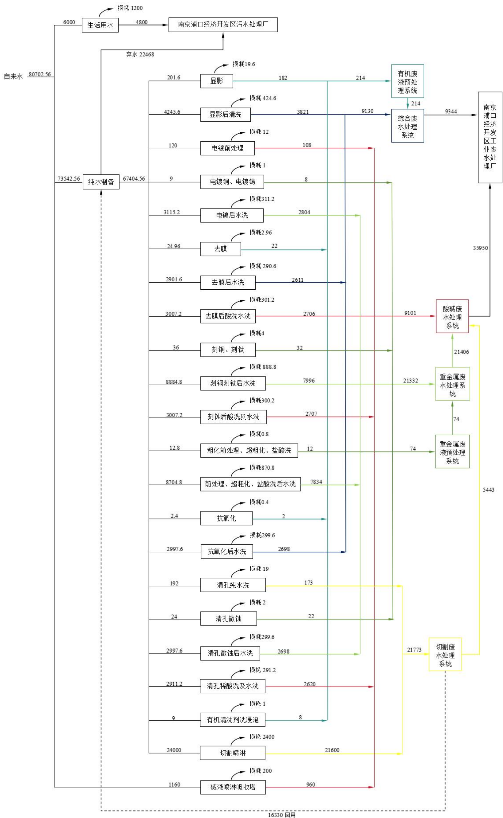
图 2-1-2 本项目水平衡 (t/a)
