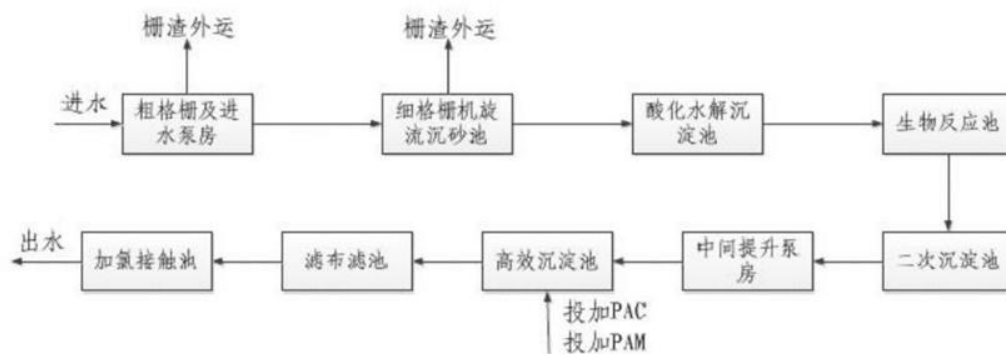
图 4-3 浦口开发区污水处理厂工艺流程图
